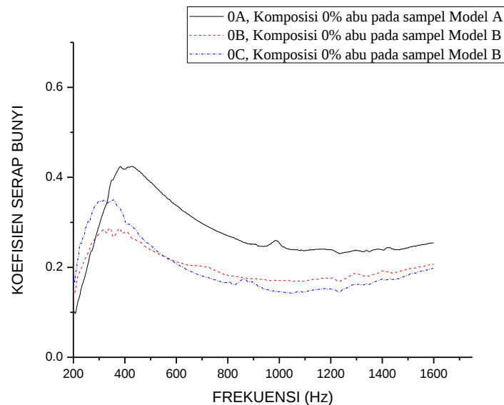
Gambar 6. Grafik koefisien serapan bunyi variasi konfigurasi Resonator Helmholtz
