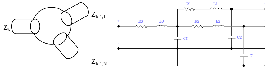
Gambar 3. Resonator Tree dan analogi listriknya
