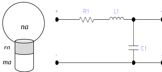
Gambar 2. Resonator Helmholtz dan analogi listriknya
