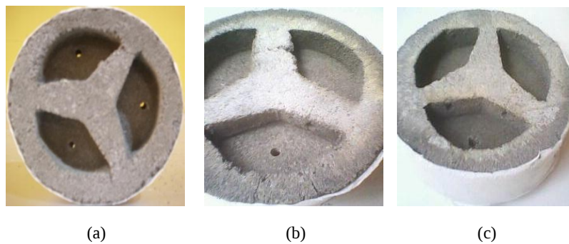
Gambar 5. Sampel batako dengan variasi posisi resonator (a) Model A, (b) Model B, (c) Model C
